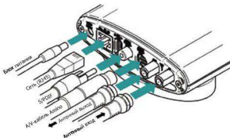
Рис. 7. Подключение приставки AmiNET110
