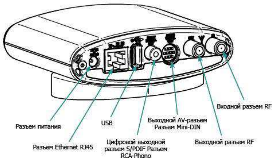
Рис. 2. Задняя панель приставки AmiNET110
