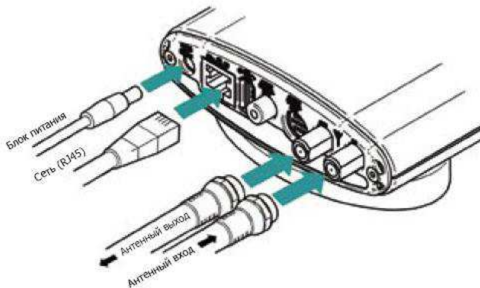
Рис. 6. Подключение приставки AmiNET110
