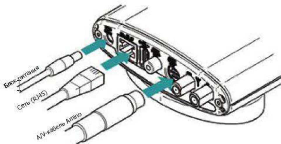
Рис. 5. Подключение приставки AmiNET110
